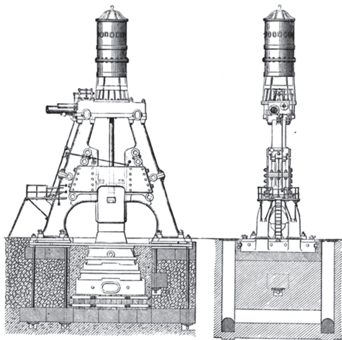
Паровой молот, созданный в 1839 году Джеймсом Несмитом (конструктивная схема и реконструкция в работе)
