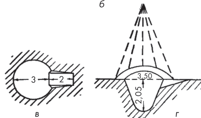
Палеолитическое жилище, обнаруженное при раскопках Тимоновской стоянки: а – план; б – продольный разрез; в – план кладовой; г – разрез кладовой
