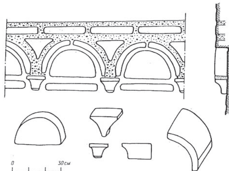
Лекальные кирпичи аркатурного пояса. Киев. Кирилловская церковь
