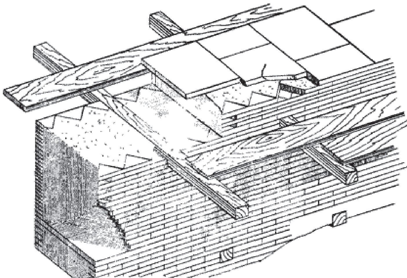
Римская бетонная стена с опалубкой-облицовкой из треугольного кирпича и поперечными связями из плоских кирпичей и деревянных брусьев (по Шуази)
