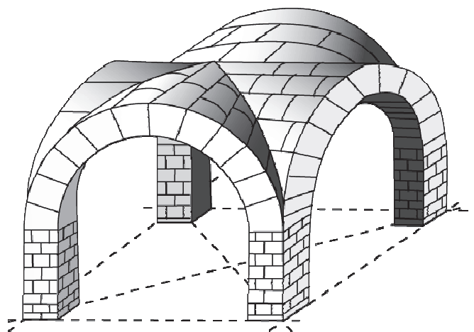
Схема крестового свода
