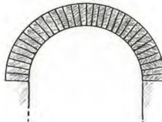
Истинная арка (швы устроены под прямым углом к линии распора)
