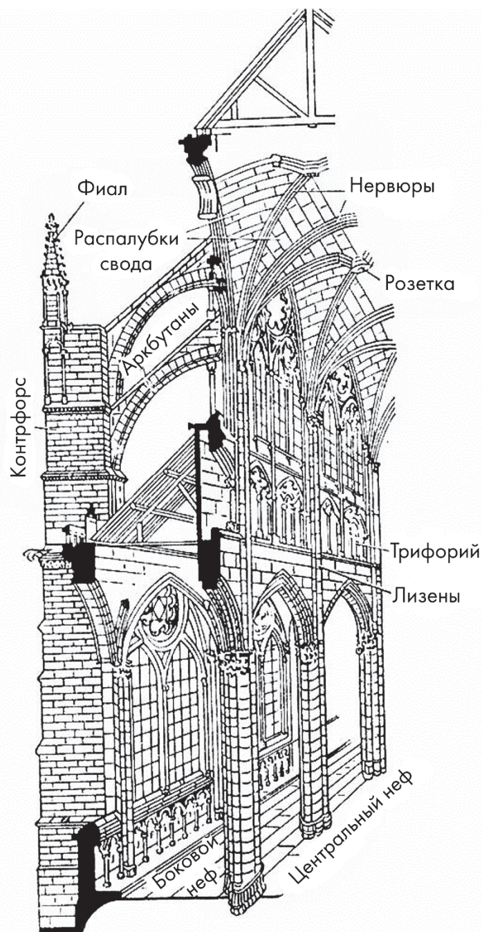
Схема стрельчатого крестового свода
