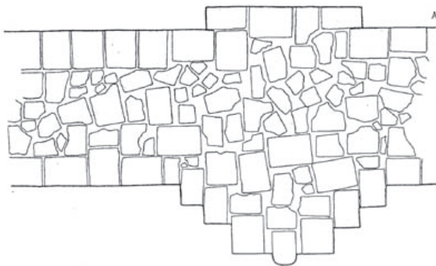
Кладка пилястры. Смоленск. Церковь на Малой Рачевке
