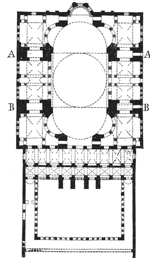
План храма св. Софии в Константинополе
