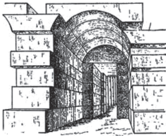
Пример ложного свода
