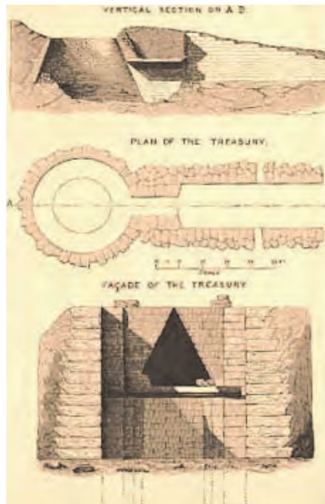
Микены. План «Сокровищницы Атрея» XIV век до н.э.
