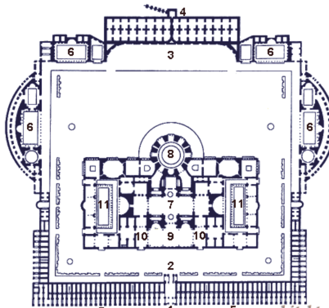
Термы Каракаллы, 206–216 годы. План. Аксонометрия:
