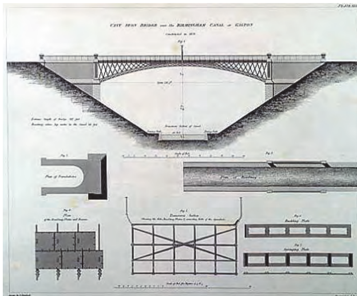
Проект моста Тельфорда
