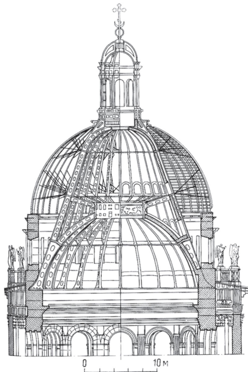
Купол Исаакиевского собора в Петербурге
